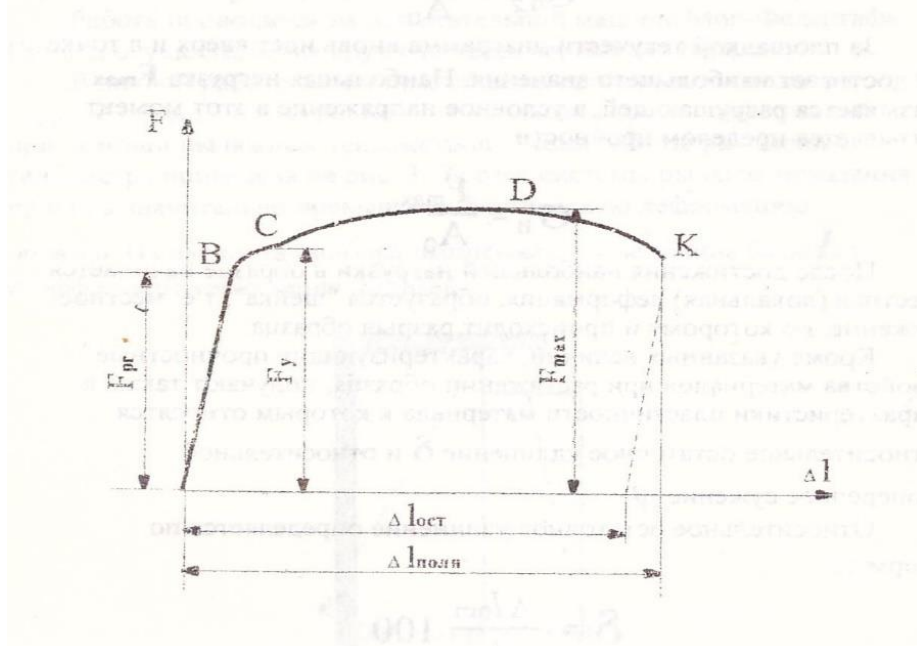
Рис. 2 Диаграмма растяжения образца из малоуглеродистой стали
