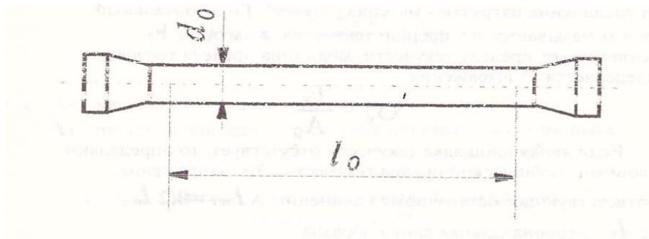
Рис. 1 Стандартный образец для испытания стали на растяжение
